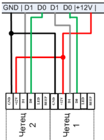
Фигура 19. Свързване четците на контролера
