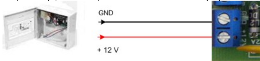
Фигура 6. Захранване
