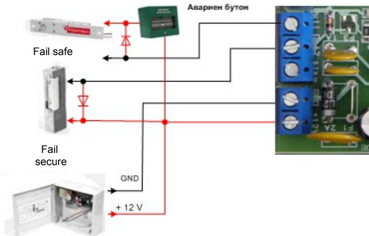
Фигура 5. Свързване на защитни диоди
